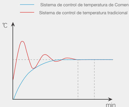
Diagrama isotérmico de la incubadora
